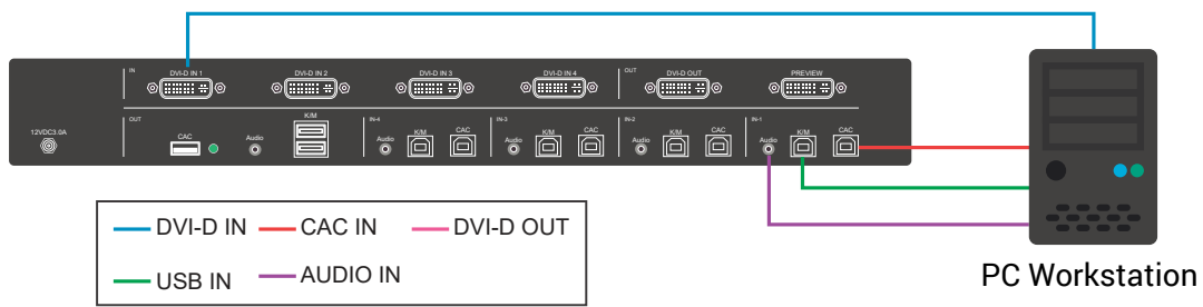
Figure 7-1: SA-DMN-DP-P
